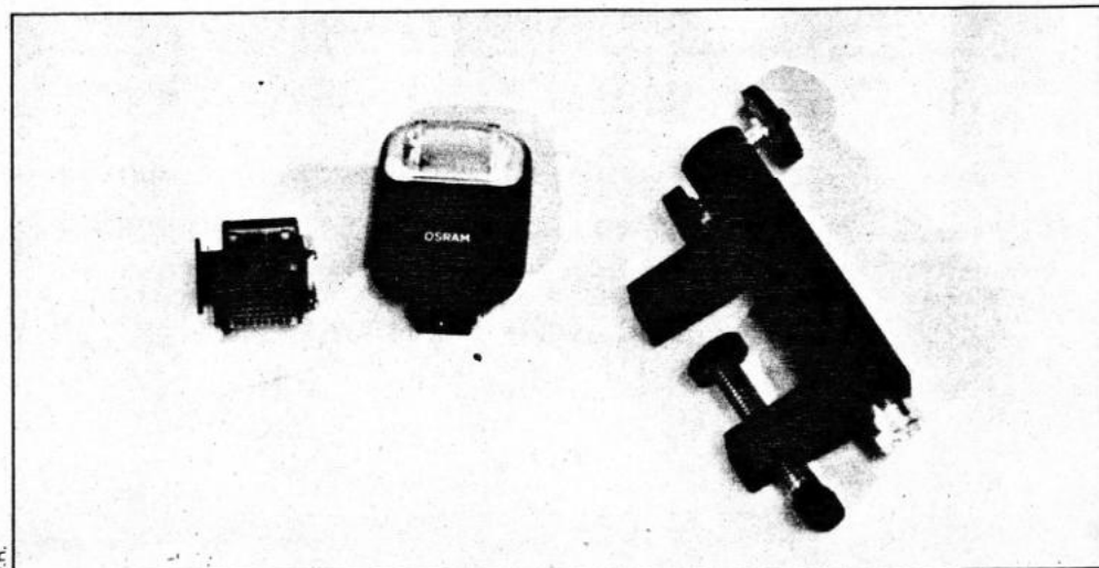
Détails de l'« antiradar »: la cellule, le flash « esclave » et son support.
